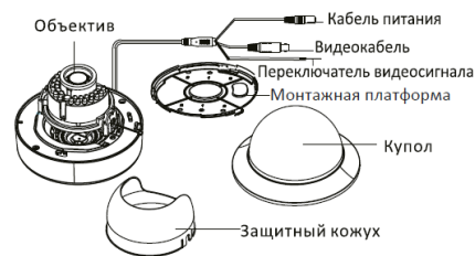
Рисунок 1-13 Купольная камера II типа
